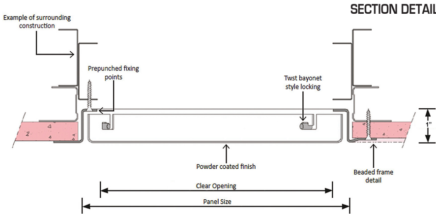
WB GP 100 Premium Access Door
